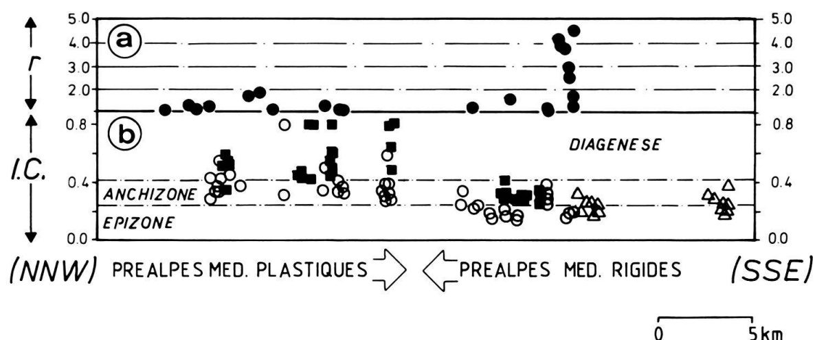
Fig. 6. Evolution de l'intensité de la déformation et du degré de métamorphisme associé en fonction de la position structurale de chaque échantillon analysé dans la nappe des Préalpes médianes. (a) intensité de déformation r = R_{xy} + R_{yz} - 1 (WATTERSON, 1968) mesurée sur des pellets; (b) cristallinité de l'illite (I.C. = index d'après KÜBLER, voir MOSAR, 1988a, b); triangles = échant. du Trias des Préalpes médianes rigides, carrés = échant. du Malm, cercles = échant. de Couches Rouges (Crétacé sup. - Tertiaire). Les limites NNW et SSE de ce diagramme correspondent aux limites de la coupe de la fig. 2.
