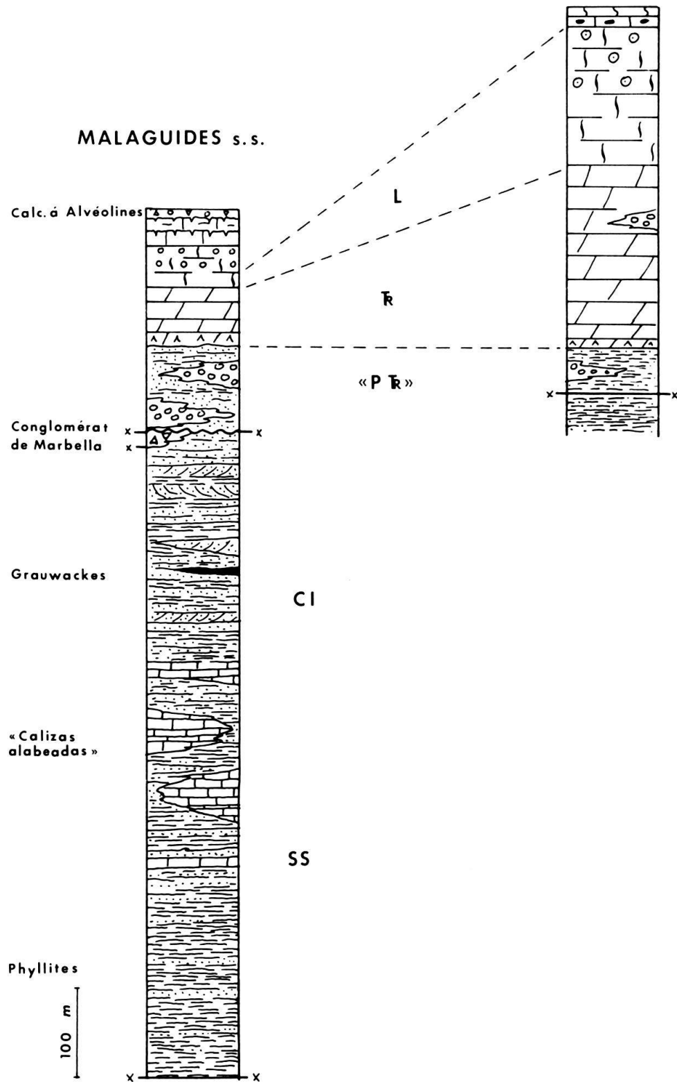
Fig.3. Coupes stratigraphiques synthétiques des Malaguides et de l'unité de Cabrilla (Dorsale interne) de la Serranía de Ronda. Indices stratigraphiques: L = Lias, R = Trias, « P R » = « Permo-Trias », CI = Carbonifère inférieur, SS = Silurien supérieur.
