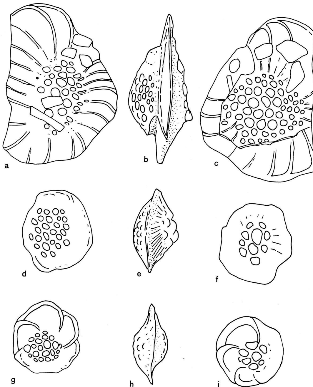
Fig. 3. Sirtina orbitoidiformis BRÖNNIMANN and WIRZ, n. sp.
