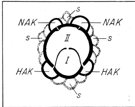
Fig. 1. Schematische Darstellung des Embryonalapparates der Lepidocyclinen . I = Initialkammer; II = Zweite Kammer des Embryonalapparates; HAK = Hauptauxiliarkammern; NAK = Nebauxiliarkammern; s = Symmetrische Interauxiliarkammern.
