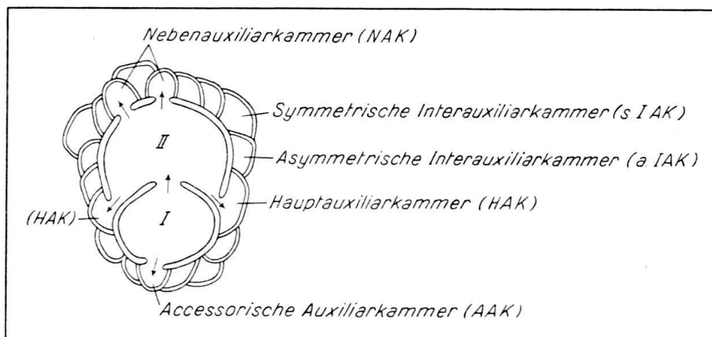
Fig. 2. Schematische Darstellung des Embryonalapparates und der periembryonalen Äquatorialkammern bei höheren Orbitoididen und Myogypsiniden. Die Pfeile geben die Stolonen zwischen den Kammern des Embryonalapparates und den HAK, NAK und AAK an. I = Protoconch, Initialkammer; II = Deuteroconch, 2. Kammer des Embryonalapparates (Aus P. BRÖNNIMANN Lit. 5).
