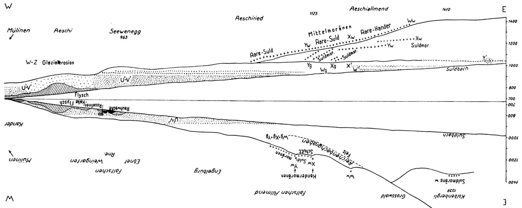
Fig. 1. Längsprofil des Suldbachgrabens, 1:25.000, auf eine Gerade projiziert.
