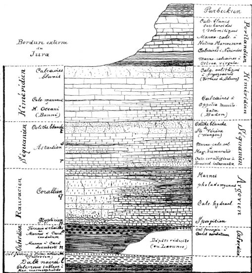
Résumé stratigraphique, Echelle 3/1000
