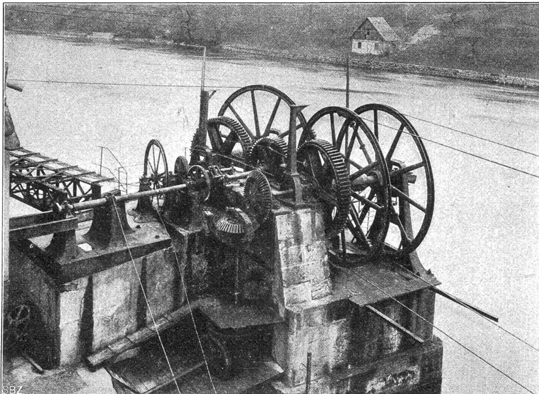
Schaffhauser Wasserwerke. Richtungsänderung und mehrfache Kraftabgabe auf Pfeiler IV.
