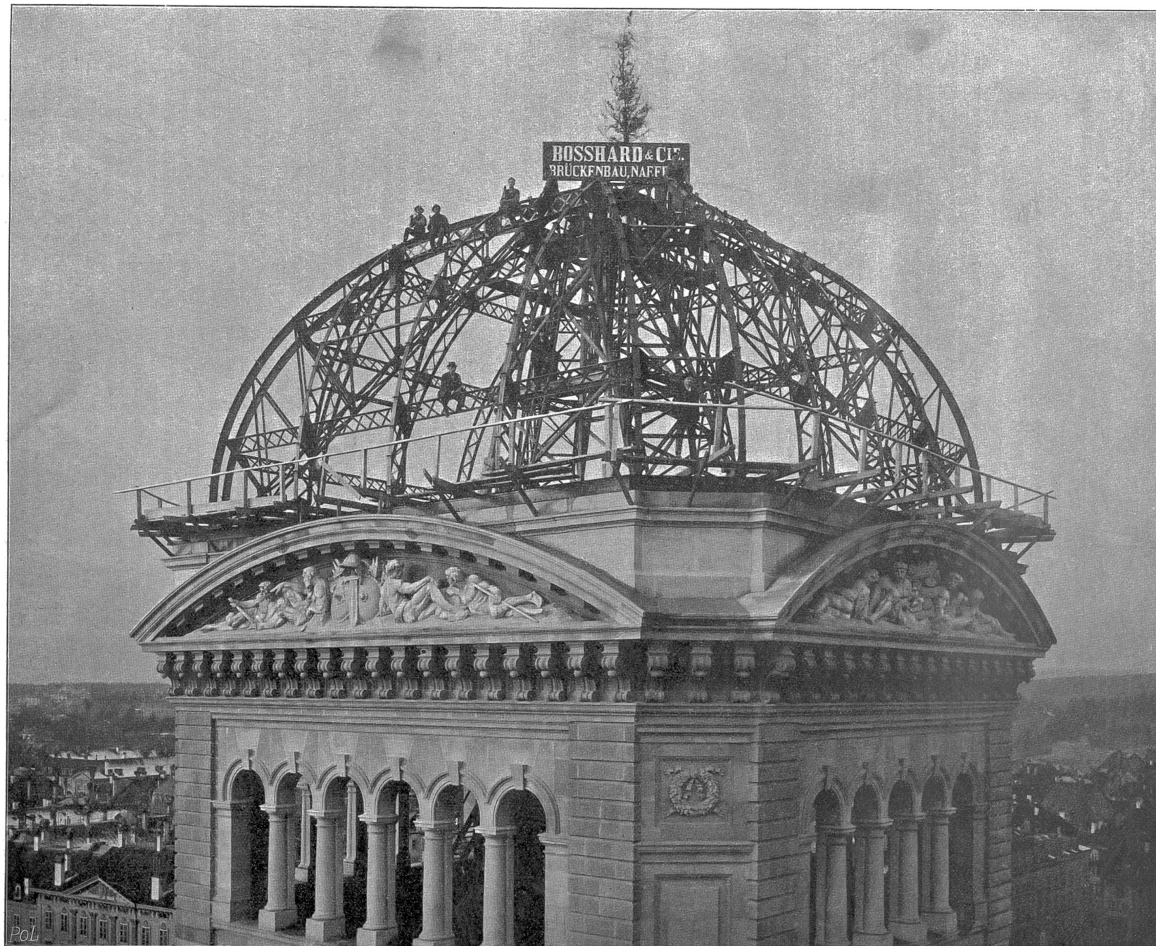
Kuppelbau am Bundespalast in Bern. Ausgeführt von Boshard & Cie, Näfels. Illustrationsprobe aus „Die Industrielle und Kommerzielle Schweiz“. (Verlag: Polygraphisches Institut A.-G., Zürich).
