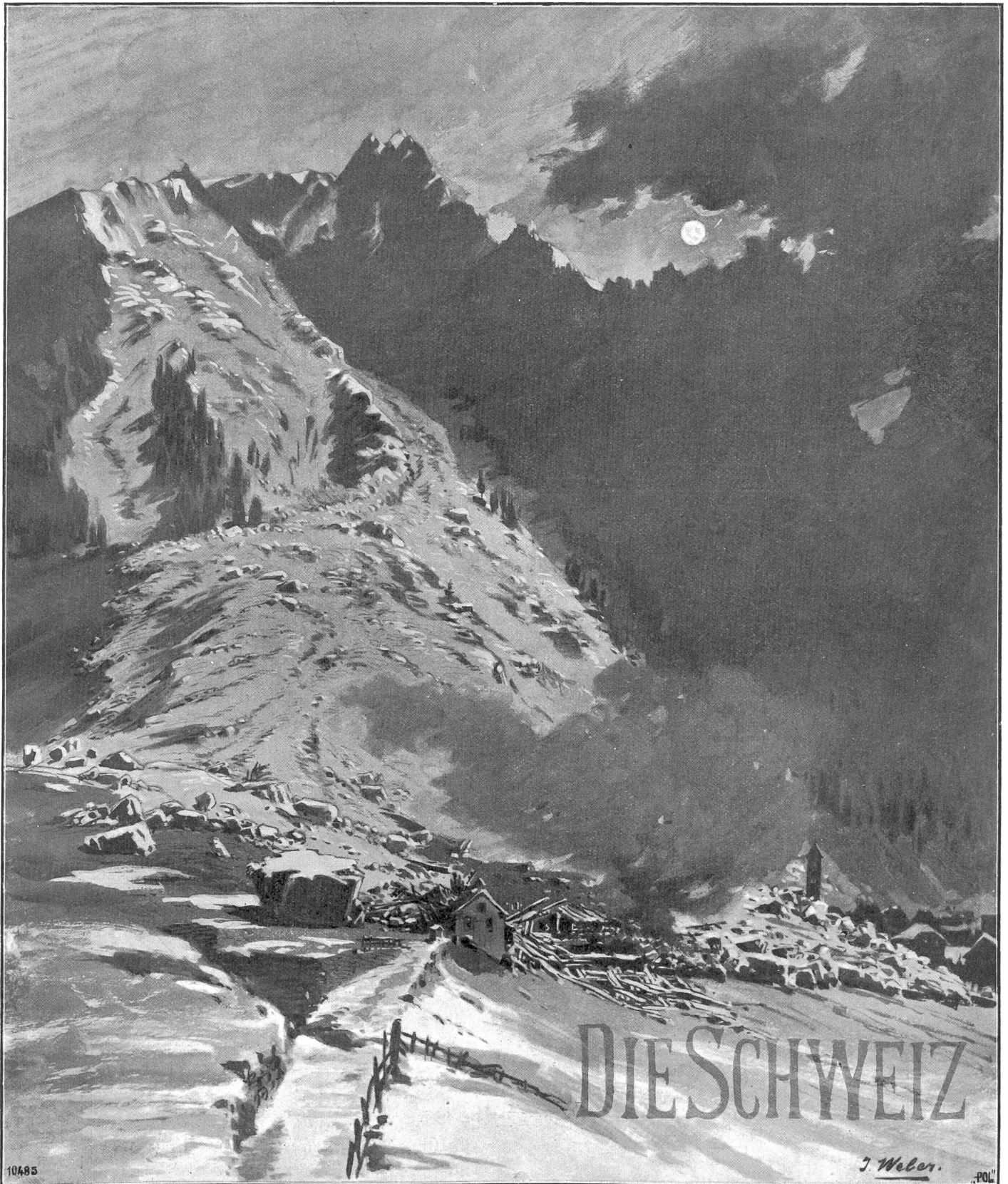
Der Bergsturz von Nivolo. Originalzeichnung nach der Natur von J. Weber, Zürich.
