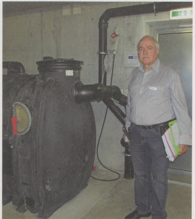
In diesem Plastiktank wird das Abwasser aus der Küche getrennt: Oben schwimmt Öl, unten fliesst Wasser ab.
