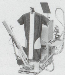
Finisher NTR. 890 für Hemden, Blusen, Schürzen, Arbeits- und Freizeitbekleidung
