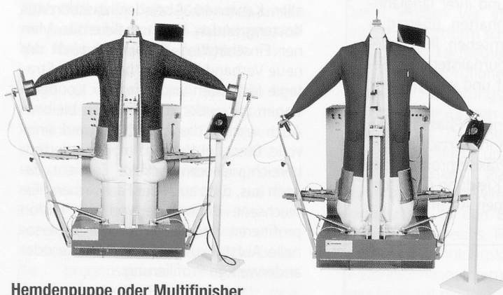
Hemdenpuppe oder Multifinisher zum Bügeln von schleuderfeuchten Hemden, Schürzen und Berufskittel. Dazu die Kragen-Manschetten-Pressse
