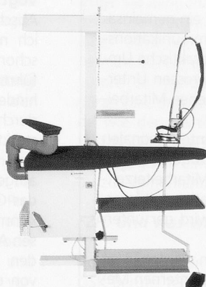
Kaltbügeltisch mit Ärmelholm • Saugen und Blasen • Beste Finishqualität • Unterdampf
