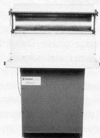
Hemdenpuppe oder Multifinisher zum Bügeln von schleuderfeuchten Hemden, Schürzen und Berufskittel. Dazu die Kragen-Manschetten-Pressse
