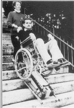
TREPPENRAUPE passend zu beliebigen Rollstühlen, für gerade Treppen
