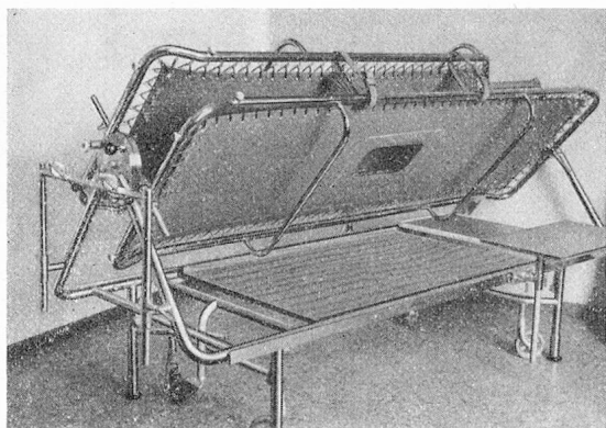
Drehbett
