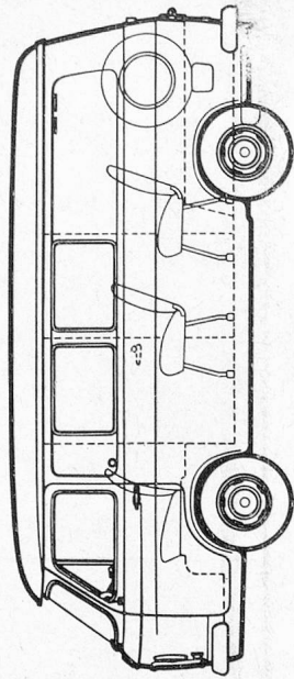
Kombi
