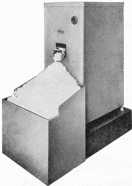
Schuppeneis-Erzeuger
