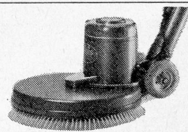
Wibis 1500 Mehrzweck-Bodenpflegemaschine
