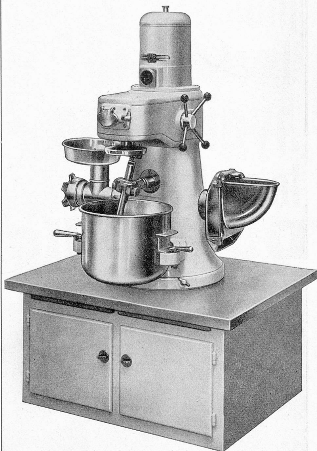
Combirex-Maschine, drehbar
