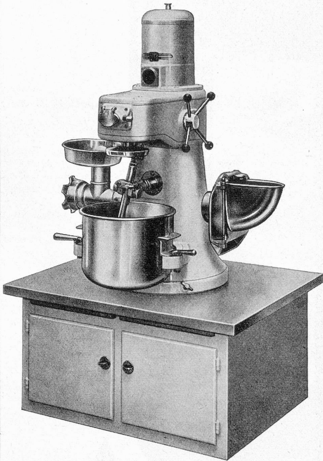
Combirex-Maschine, drehbar
