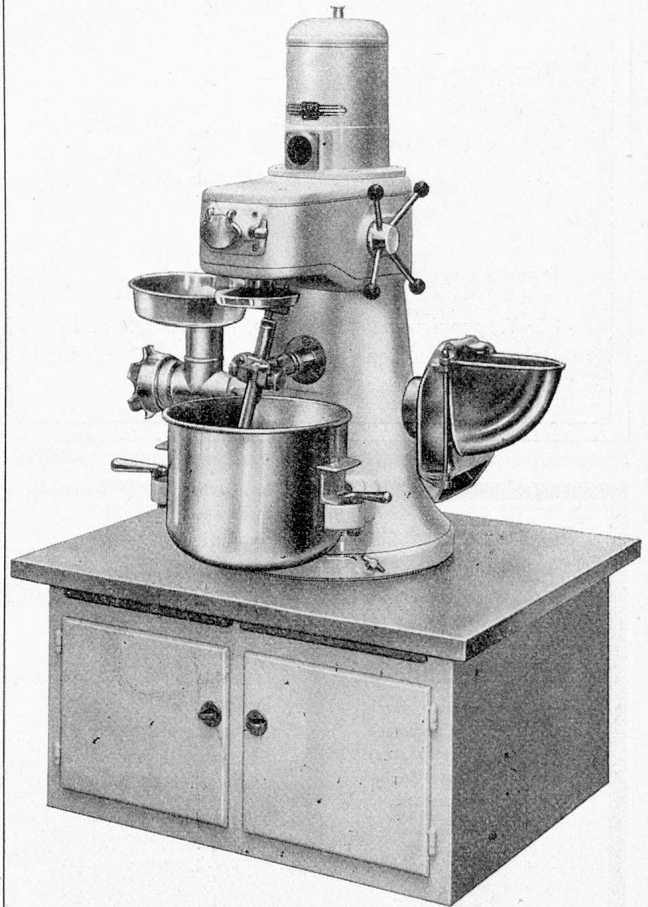
Combirex-Maschine, drehbar
