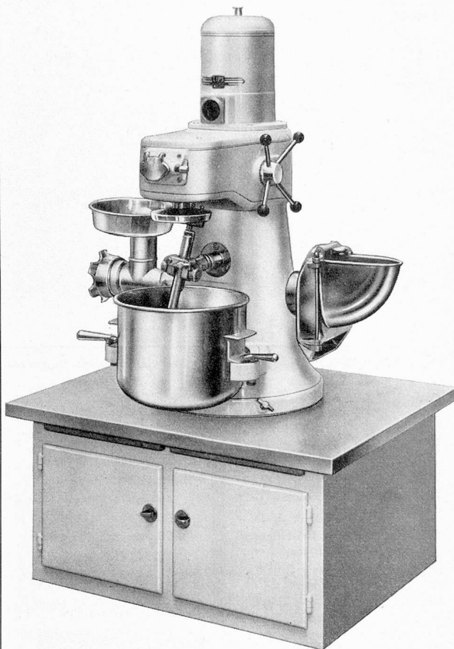
Combirex-Maschine, drehbar
