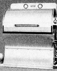
Type I
