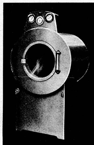
Wäsche-Tumbler (Wäschetrockner) 45 kg Trockenwäsche pro Stunde
