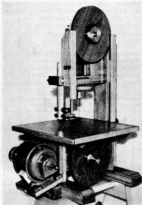
Bandsäge
