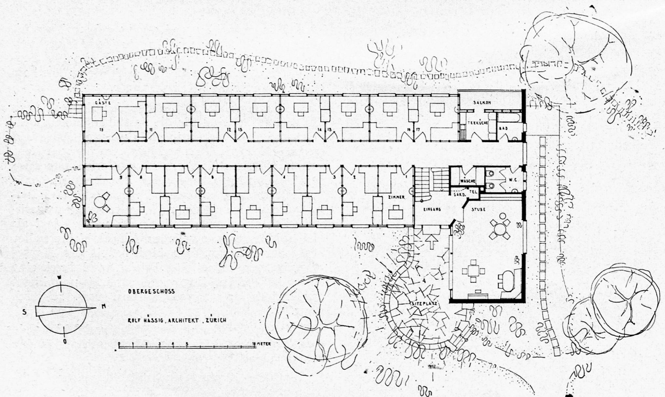
Abb. 4: Obergeschoss
