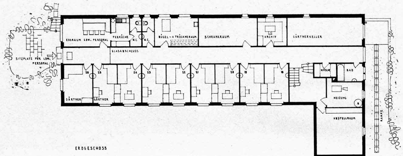
Abb. 3: Erdgeschoss
