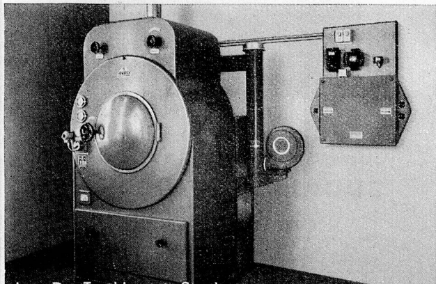
Avro-Dry-Tumbler mit Sterilisator Total-Anschlussw. 28 kW in der Heil- und Pflgeanstalt Rosegg Solothurn AVRO 4809
