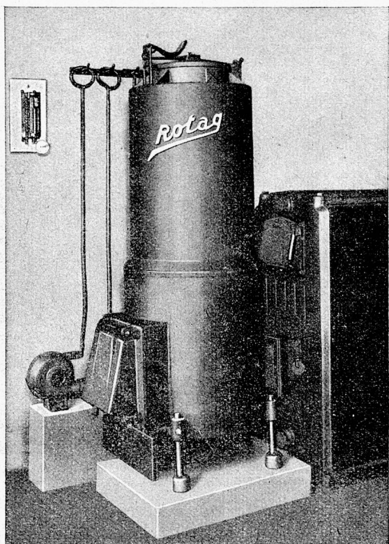
„ROTAG“-Vorbaubrenner
