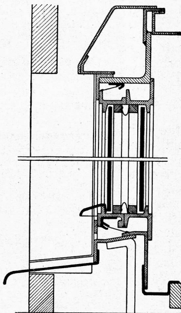
Fig. 2 Eisenfenster, doppelvergl., SUPERHERMIT in Halteprofil D-2 u. D-4. Ausführungen: Universität Basel, Theodor-Stranum (Operationssaal) Zürich. Ausführung in Einfachverglasung: Fabrikneubau Landis & Gyr, Zug, Schweizer Sender Schwarzenburg, Bäckereineubau des Konsumvereins Zürich, etc.
