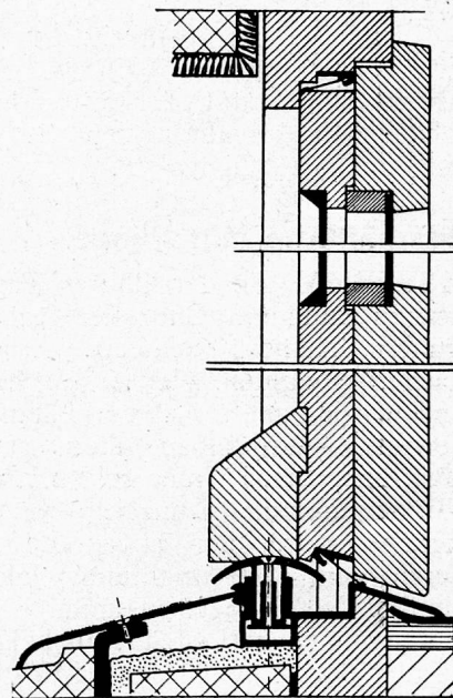
Fig. 3 Balkontüre, doppelvergl., SUPERHERMIT in Halteprofil D-2, kombiniert mit Spezialschwelle O-11/13 für Spitäler, Sanatorien etc. Ausführung: Kantonsspital Chur.
