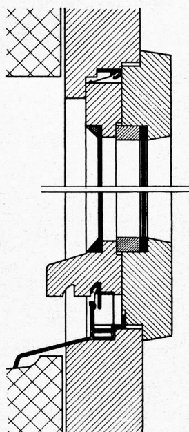
Fig. 1 Holzfenster, doppelvergl., SUPERHERMIT in Halteprofil D-2 und D-3, kombiniert mit Regenprofil O-10. Ausführungen: Kantonsspital Chur, Frauenspital St. Gallen, Bethesda-Spital Basel, Kinderspital Zürich.
