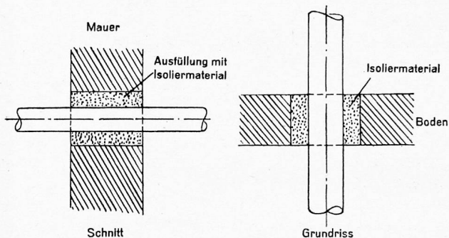
Abbildung 4 Beispiele für Mauer- und Bodendurchführungen
