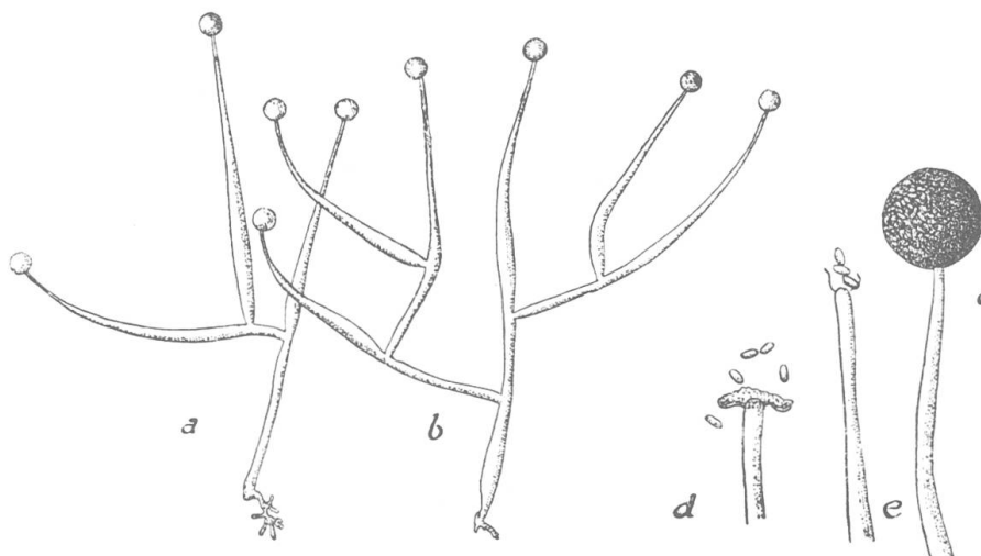
Fig. 56. Mortierella Bainieri .
