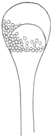
Fig. 14. Columelle infundibuliforme.
