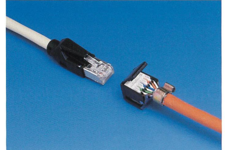
Bild 2. Bei der Kategorie 6 ist kein «Mix und Match» mehr möglich.
