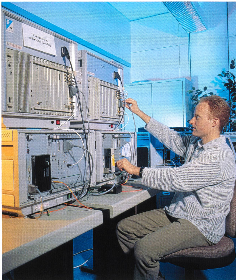
ATM-Terminal-Adapter für TV Distribution. Die ATM-Terminal-Adapter (Empfänger) wandeln die ATM-Zellen in analoge Signale (Fernsehsignale) um. Sie sind netzseitig an die ATM-Plattform und anschlussseitig am Fernseher angeschlossen. Oben: Video-Decoder, unten: ATM-Terminal-Adapter (Empfänger).
