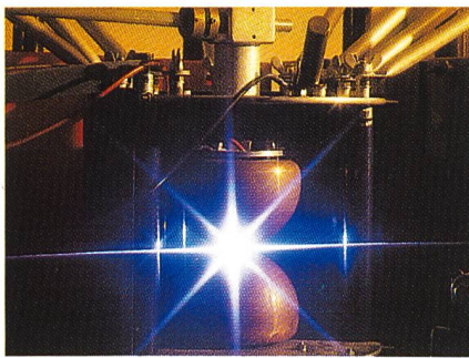
Die Blitzstoss-Stromanlage der Direktion Forschung und Entwicklung der Telecom PTT in Ostermundigen: Ein Blitz wird simuliert, um dessen Einflüsse zu studieren.
