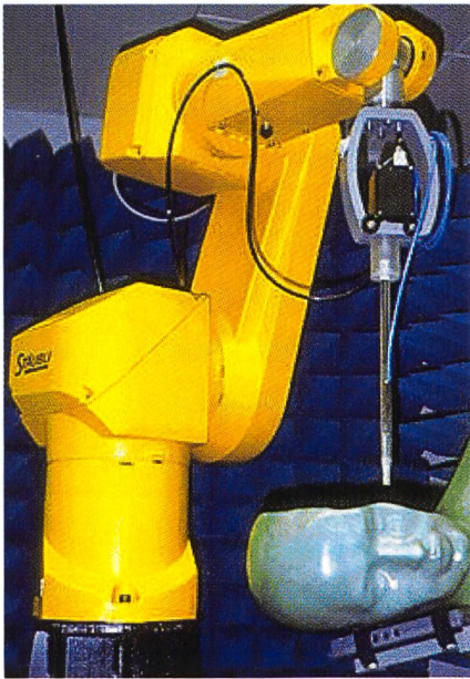
Fig. 1. Robot de mesure avec sonde triaxiale (en haut). Mannequin rempli d'un liquide comparable aux tissus humains et radiotéléphone appliqué à la tête (en bas).
