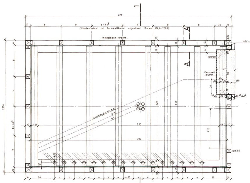
Bild 4. Grundriss.
