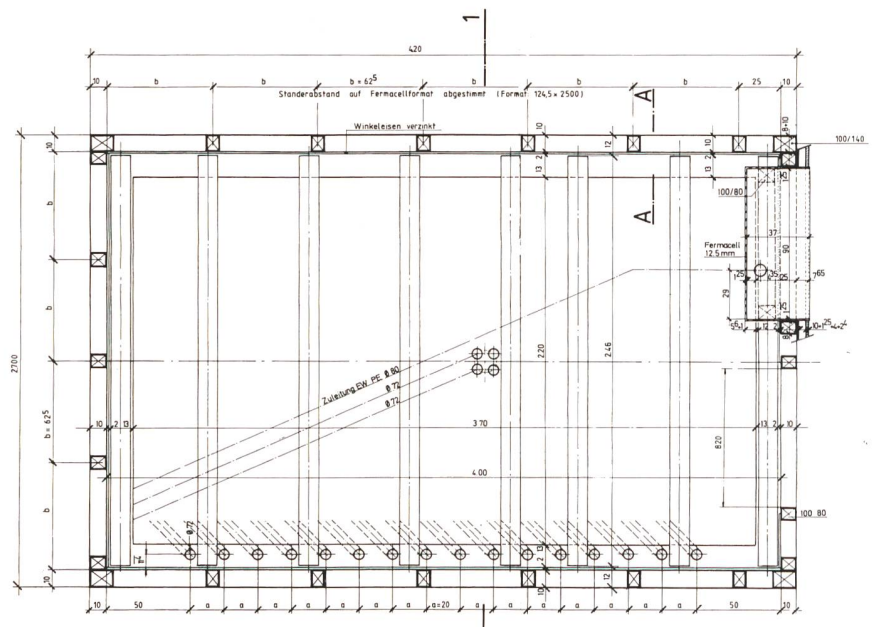
Bild 4. Grundriss.
