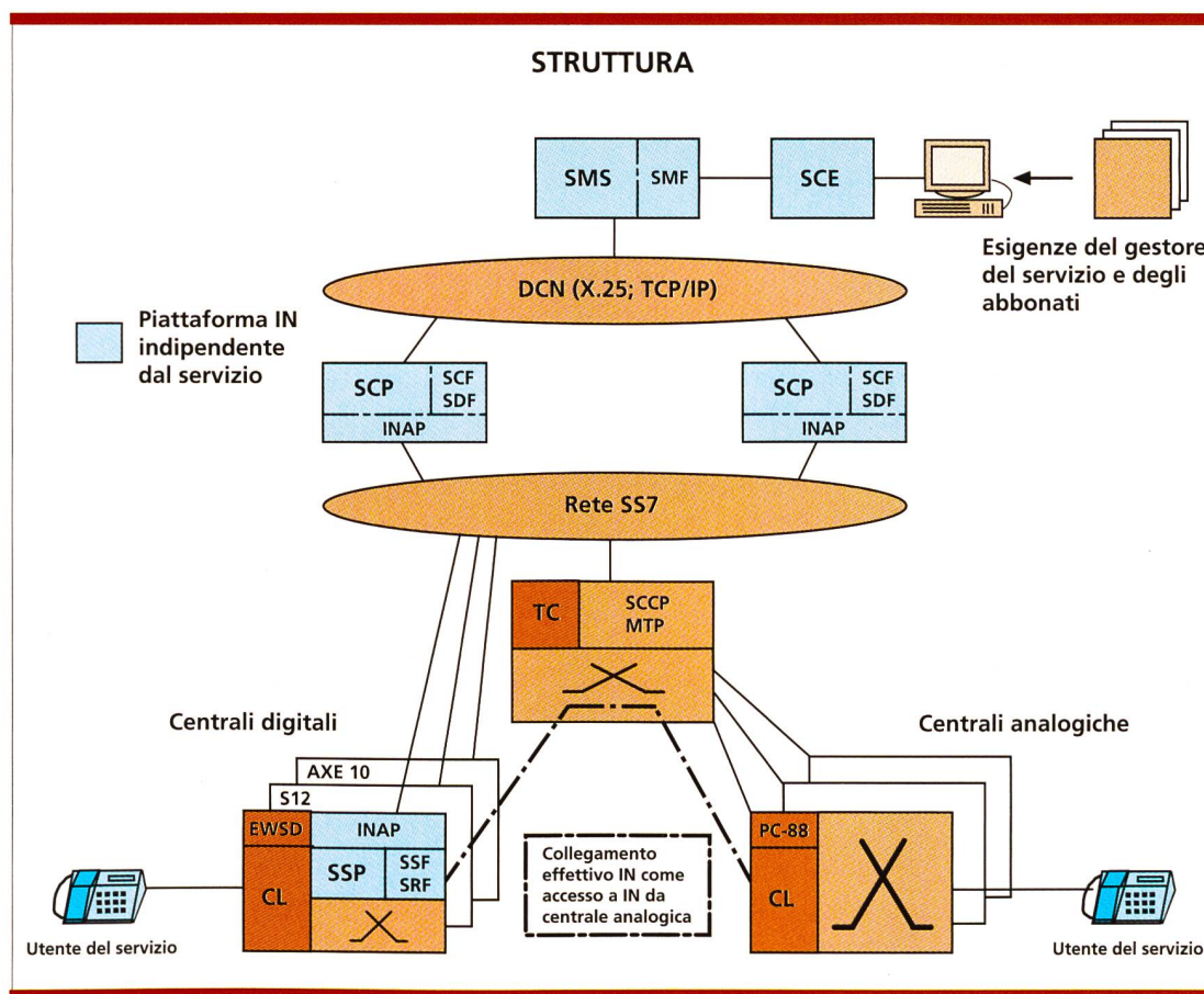
Fig. 1. Principi di funzionamento di diversi collegamenti.
