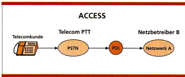
Bild 2. Die Telecom PTT ermöglicht seinem Kunden A den Zutritt zu den Dienstleistungen des Netzbetreibers B.
