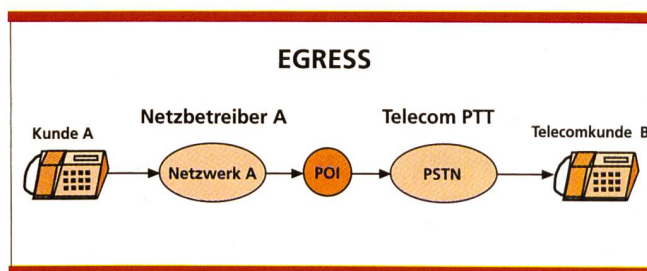
Bild 1. Die Telecom PTT terminiert den Verkehr des Netzbetreibers A zu seinem Telekomkunden B. POI: Point of Interconnection (z. B. Eingang oder Ausgang der Transitzentrale); Netzbetreiber: Drittfirma, die eine Konzession für den Betrieb eines Netzes besitzt; Netzwerk: eigenes oder mit Mietleitungen aufgebautes Netzwerk, das die Vermittlung und Übertragung von Informationen ermöglicht; Kunde A, B: Endkunde, der ein Endgerät in Form eines Telefon-, Fax- oder Datenübertragungsgerätes betreibt.
