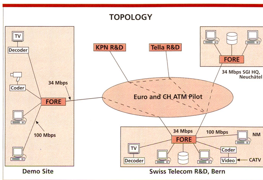
Bild 2. Topologie der Plattform ATM Corporate Networks
