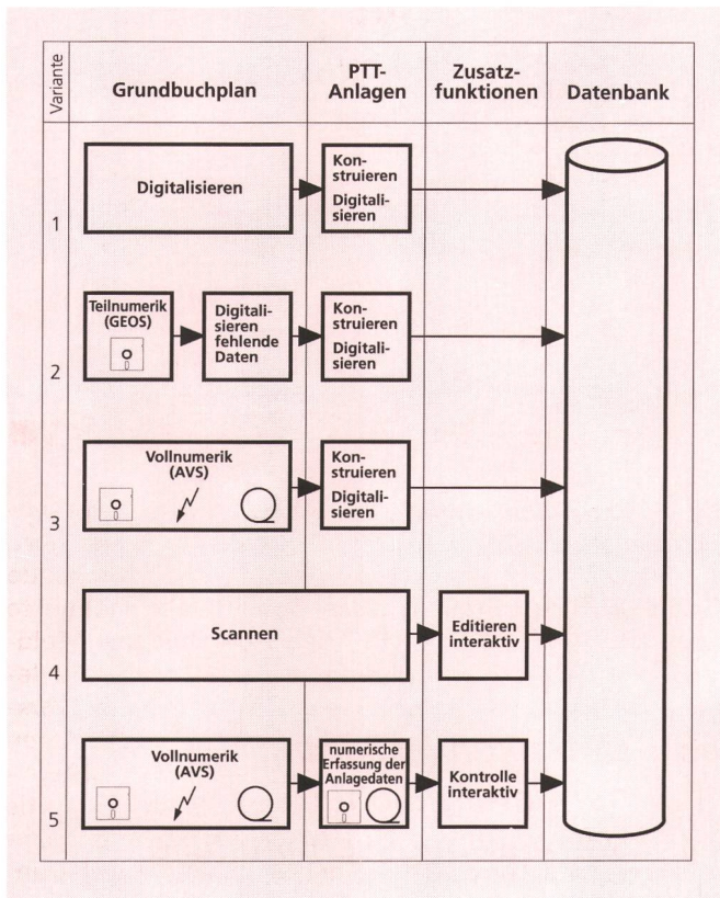
Fig. 2 Datenübernahme – Varianten für Situationsplan AVS Amtliche Vermessungsschnittstelle
