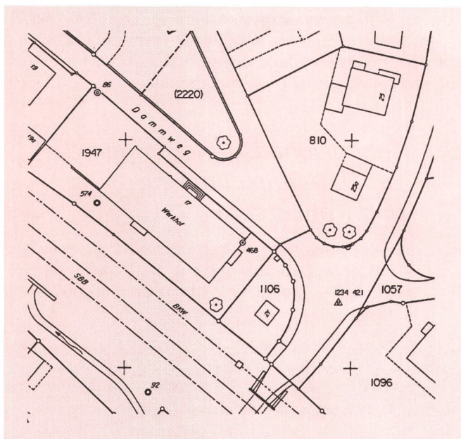
Fig. 4 Grundbuchplan als Grundlage für den Werkleutungsplan
