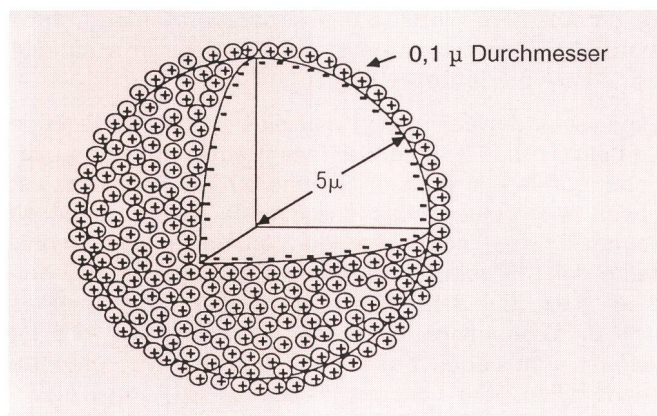
Fig. 6 Ionenaustauscher-Partikel – Particule de l'échangeur d'ions Durchmesser – Diamètre
