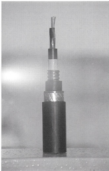
Fig. 2 Kabelaufbau
