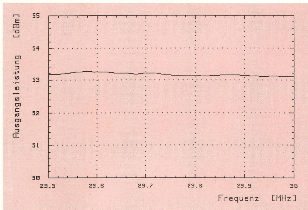
Fig. 3 Typische Mess- ergebnisse der TL 30020 im Fre- quenzbereich Koper- nikus – Résultats de mesure typiques pour le tube TL 30020 utilisé dans la bande de fré- quences du satellite Kopernikus Ausgangsleistung – Puissance de sortie [dBm] Frequenz – Fré- quence [MHz]
