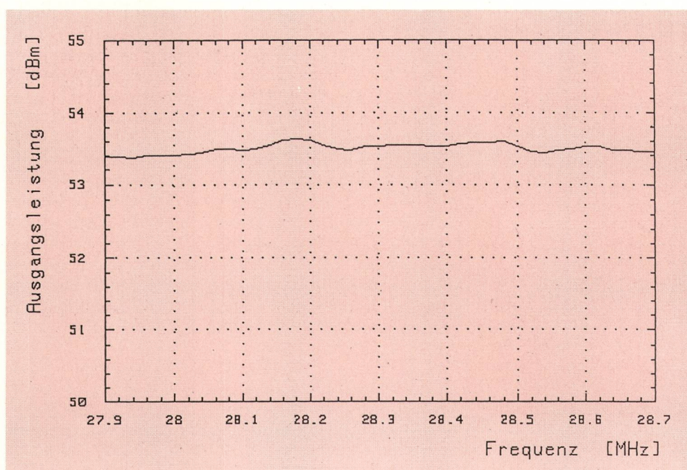
Fig. 4 Typische Mess- ergebnisse der TL 30020 im Fre- quenzbereich Olym- pus – Résultats de mesure typiques pour le tube TL 30020 utilisé dans la bande de fré- quences du satellite Olympus Ausgangsleistung – Puissance de sortie [dBm] Frequenz – Fré- quence [MHz]
