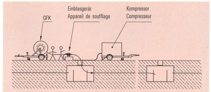
Fig. 8 Einblasdisposition – Disposition des appareils pour le soufflage
