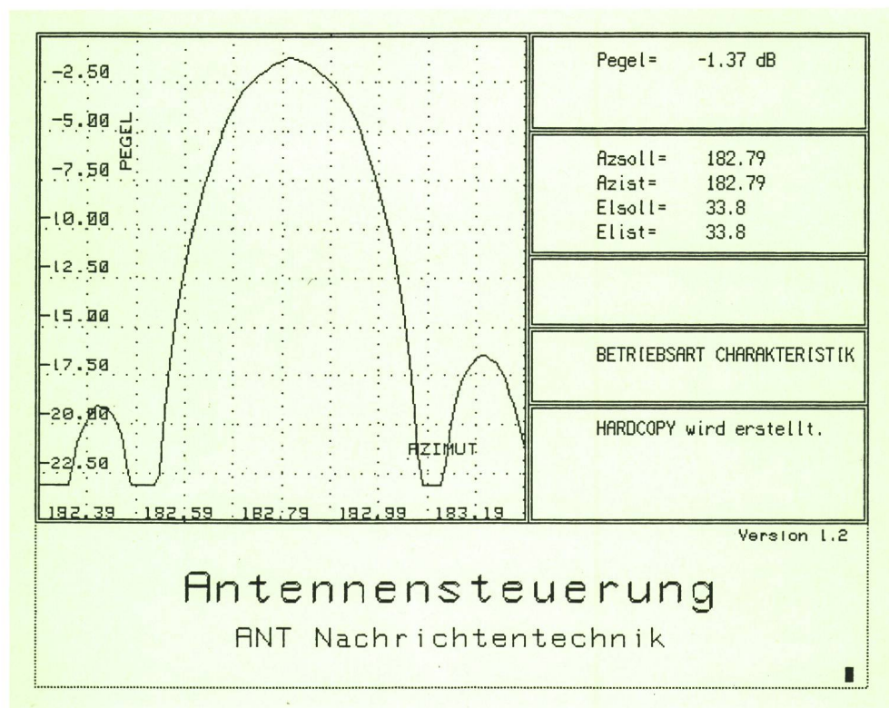
Fig. 2 Antennencharakteristik – Caractéristiques d'antenne Pegel – Niveau Azsoll – Valeur angulaire nominale en azimut Azist – Valeur angulaire réelle en azimut Elsoll – Valeur angulaire nominale en élévation Elist – Valeur angulaire réelle en élévation Betriebsart Charakteristik – Genre d'exploitation caractéristiques Hardcopy wird erstellt – Impression en cours
