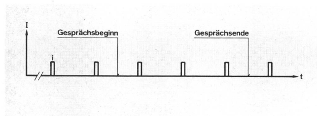
Fig. 1 Zählimpulsreihe mit zufälligem Gesprächsbeginn
