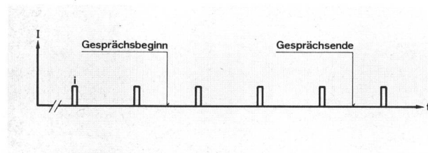
Fig. 1 Zählimpulsreihe mit zufälligem Gesprächsbeginn I Stromstärke t Zeit i Zählimpuls
