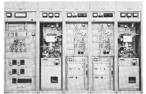
2-kW-TWT/Tetroden-Sender für Band IV/IV, Doppelausführung, passive Reserve
