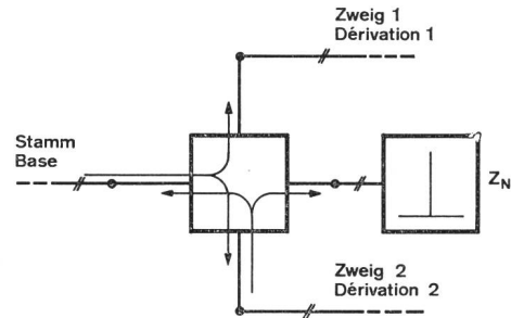
Fig. 2 Gabelschaltung - Connexion avec transformateur différentiel
