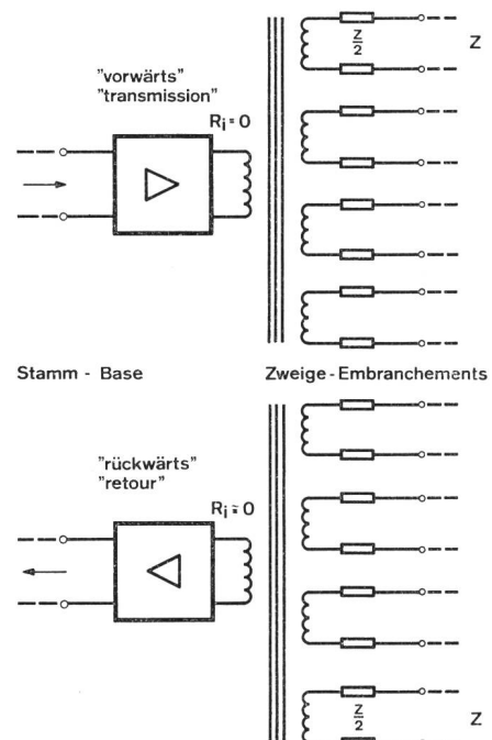
Fig. 3 Abzweigschaltung mit Verstärker - Circuit découplage avec amplificateur
