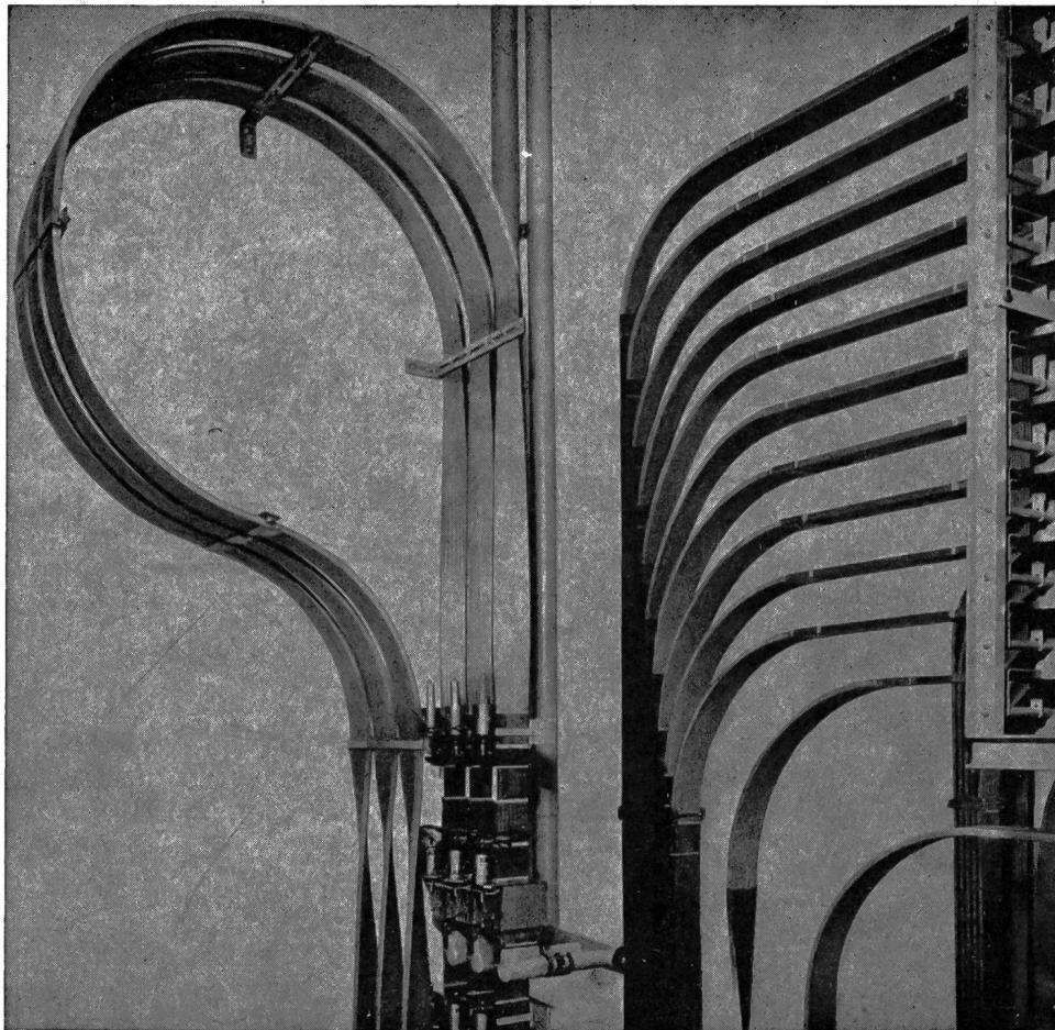
Eingangsausrüstung einer vollautomatischen Zettelrohrpost-Welchenzentrale
