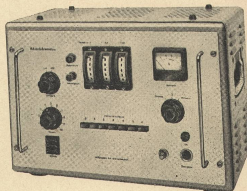
Réverbéromètre, Type B-710 Nachhallzeit-Messer, Typ B-710
