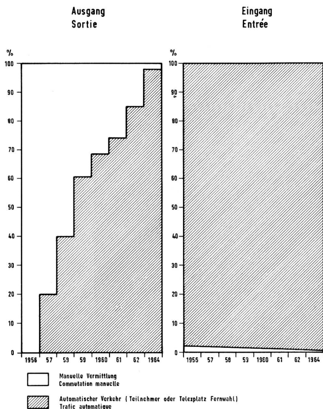
Fig. 12. Stand der Automatisierung im Telexverkehr mit dem Ausland
